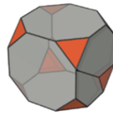
Afgeknotte Kubus
