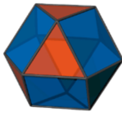
Cubo-Octaëder
