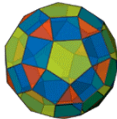
Kleine Romben-Icosidodecaëder
